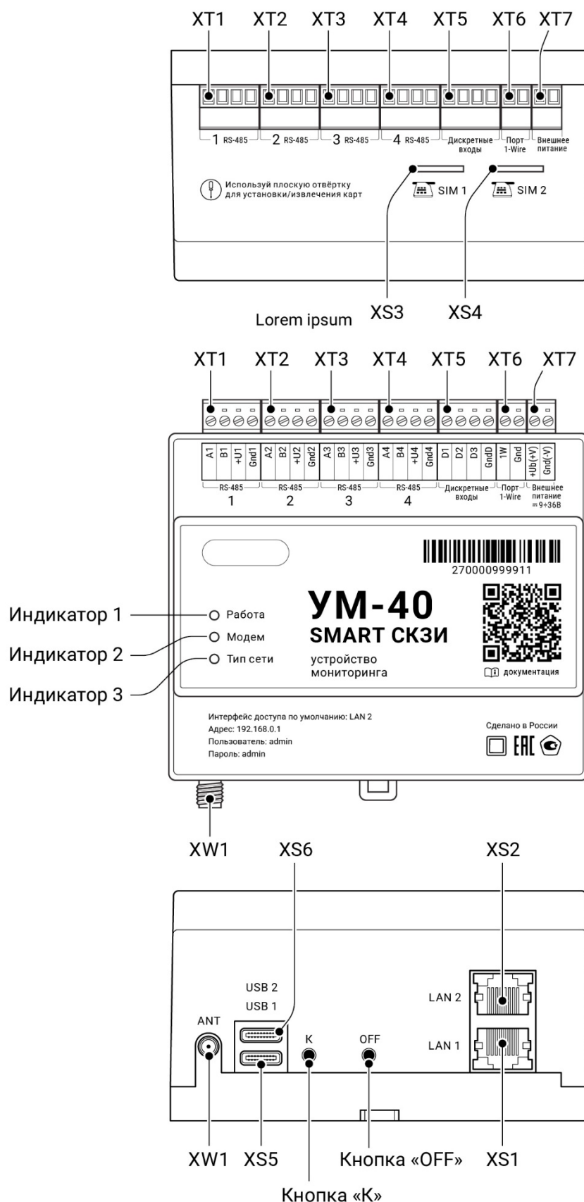
Рисунок 3 – Расположение разъёмных соединителей, индикаторов и кнопок
