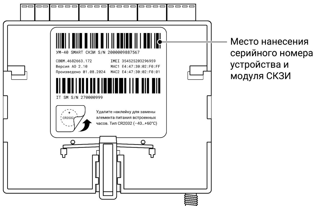
Рисунок 4 – Задняя сторона УМ
