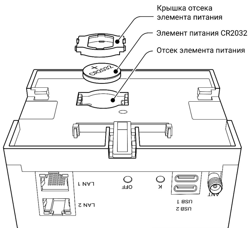
Рисунок 5 – Замена элемента питания
