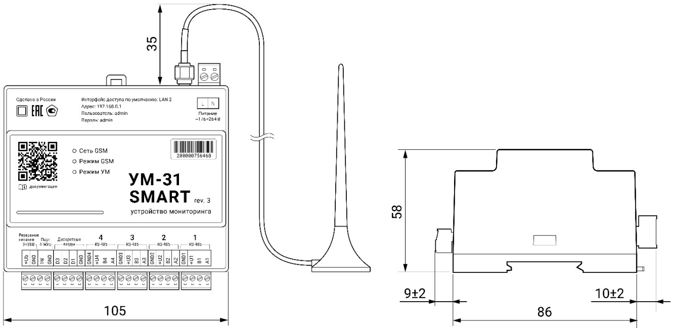
Рисунок 3 – Габаритные размеры УМ
